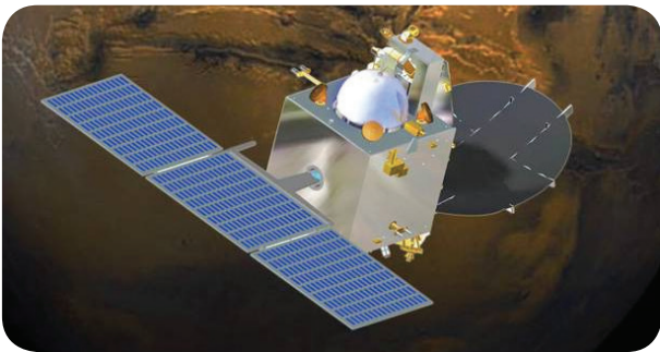
படம் 8.7 மங்களாயான்
