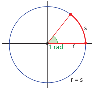
படம் 1.7 ரேடியன்
