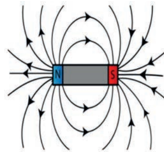
படம் 7.4 காந்தப்புலம்
