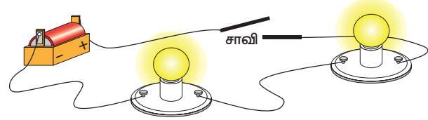
படம் 5.13 தொடரிணைப்பு
