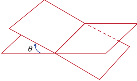
படம் 1.6 தளக்கோணம்
