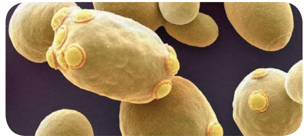
படம் 17.6 ஈஸ்ட்
